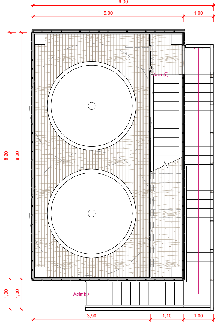
3 PAVIMENTO 02 1 : 75
